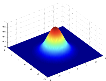
Figure – Densité d'une gaussienne isotrope \mathcal{N}(0, \sigma^2 \text{Id}_2)
