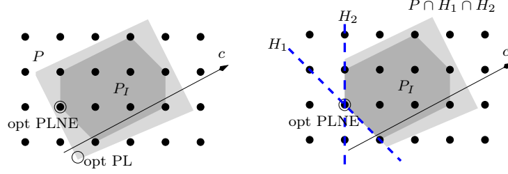
FIGURE 7.1 – Un polyèdre P (quadrilatère gris clair) et sa clôture entière P_I (hexagone gris foncé). L’optimum du programme linéaire en nombre entiers (opt PLNE) est comparé à l’optimum de son relâché continu (opt PL), pour le coût x \mapsto c \cdot x . L’ajout de deux coupes d’intégrité (demi-plans H_1 et H_2 ) conduit à un problème de minimisation sur un nouveau polyèdre (pentagone), qui redonne l’optimum du PLNE (figure de droite).
